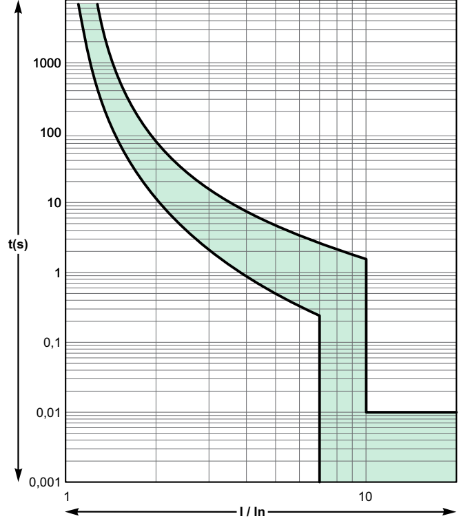
C eğrisi
