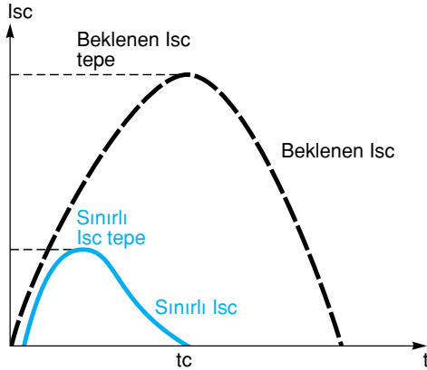
Beklenen akım ve gerçek sınırlı akım.
