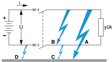
Şekilde bir IT sisteminde negatif kutup üzerinde ikinci hatası (D) olan bir kaynak gösterilmiştir.
