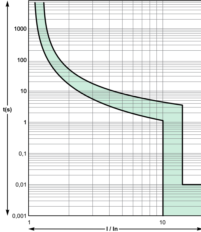
D eğrisi
