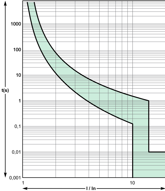
D eğrisi
