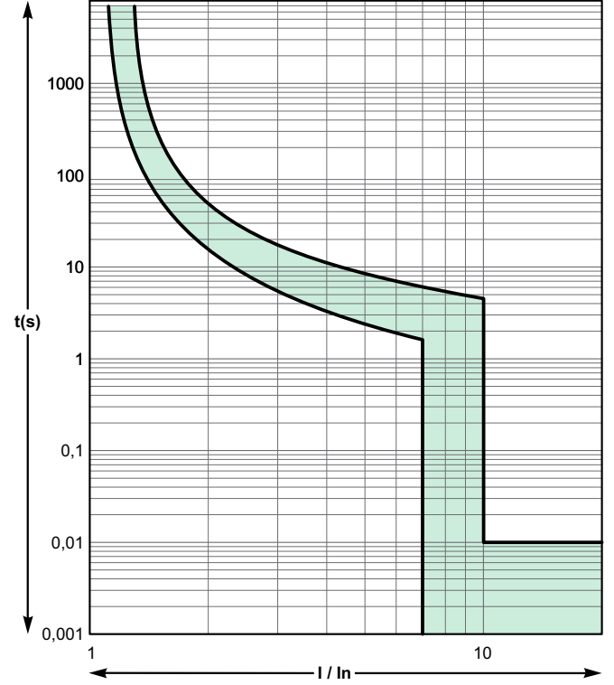
C eğrisi
