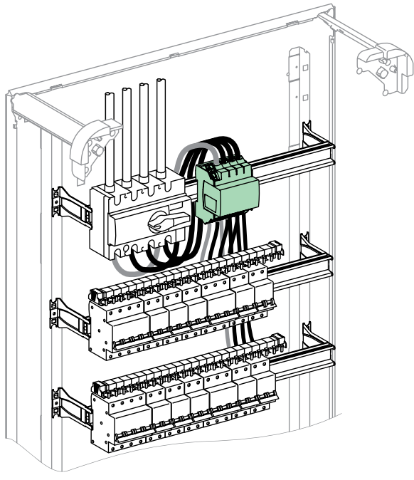
Üstten dağıtım.
